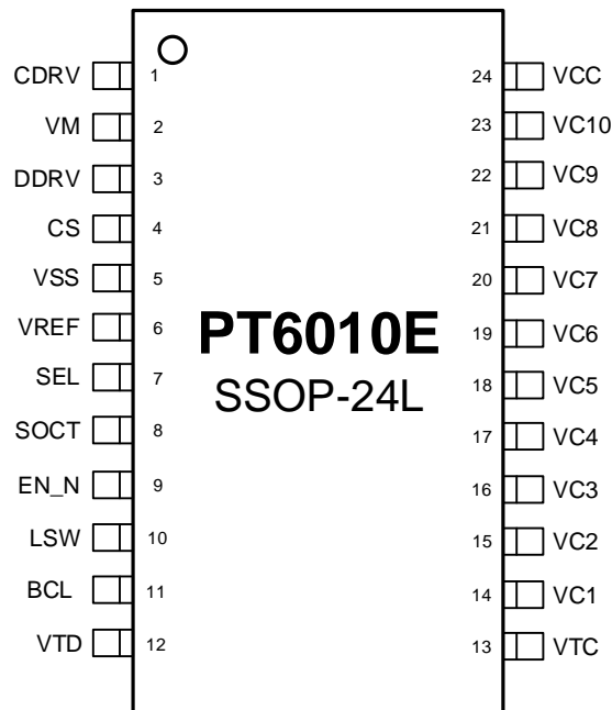
图 5. 管脚定义图
