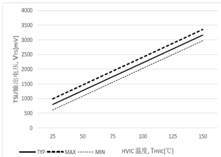
V_{TS} 电压的温度特性
